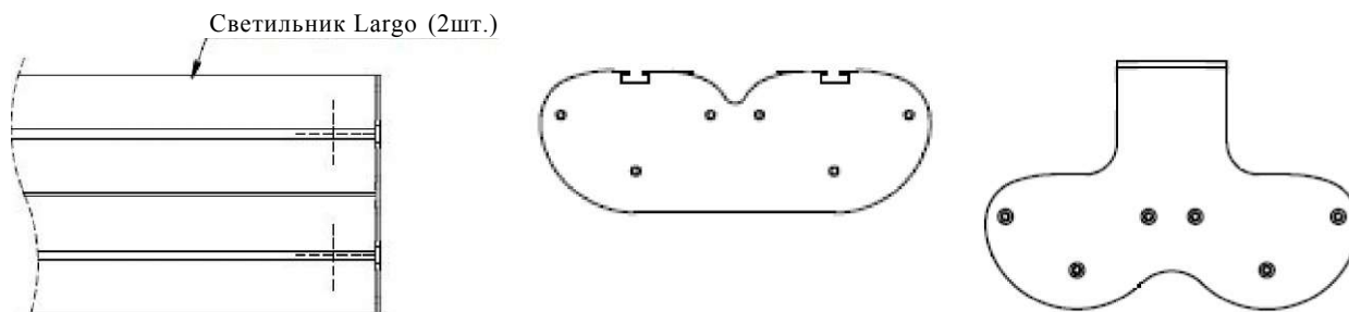
Рисунок 8 - Двойное крепление с крышкой для подвешного и с крышкой для потолочного монтажа.
