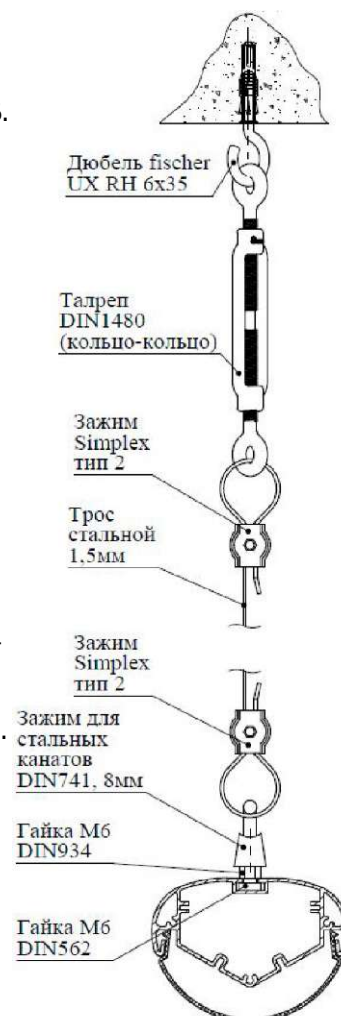
Рисунок 6 - Подвес светильника.
